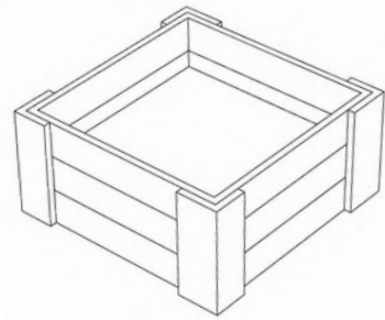
H-01 HUERTO CUADRADO
