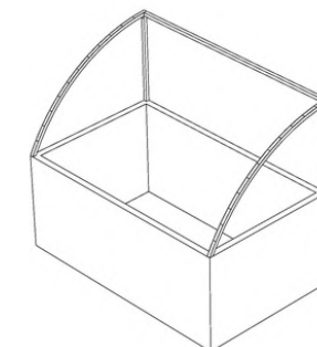
H-12 CON ESTRUCTURA GAJO Para instalar malla sombra, se sugieren especies altas en la parte posterior y bajas al frente
